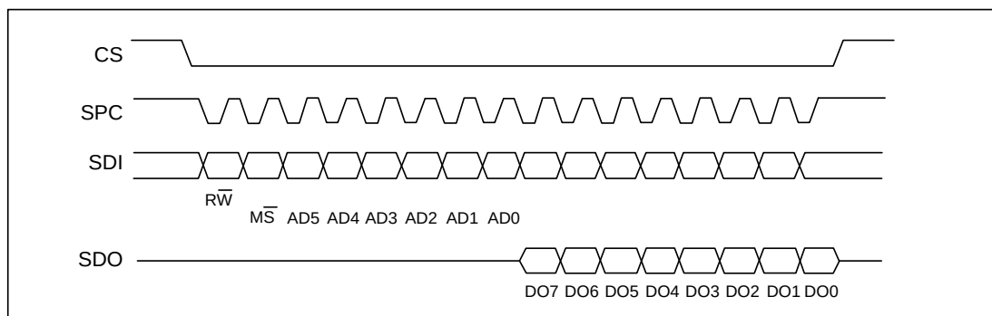
SPI读协议
