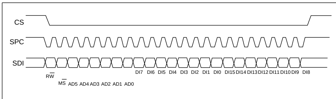
SPI多字节写协议（2字节为例）
