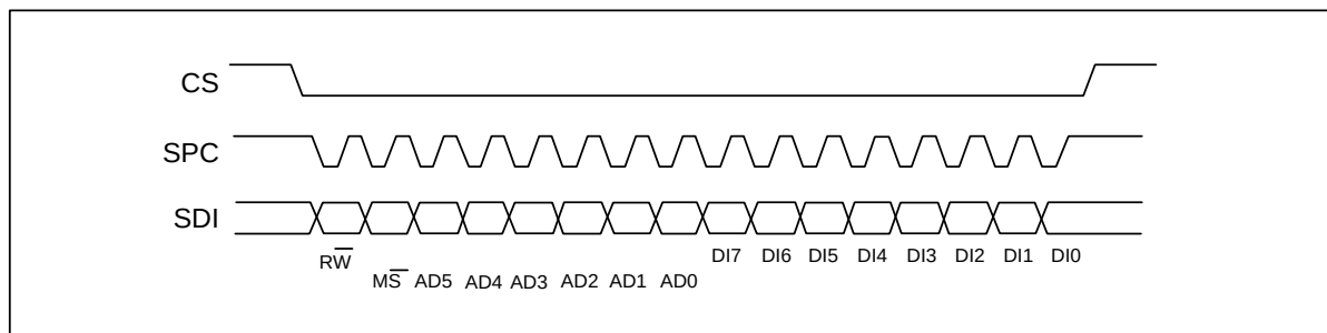
SPI写协议
